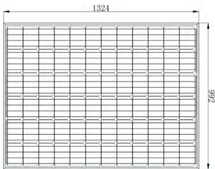
正面图
