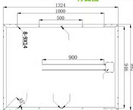
背面图
